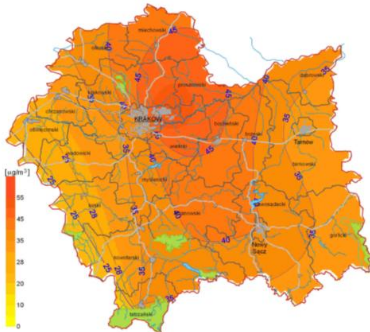
Rysunek 23. Rozkład stężeń pyłu \text{PM}_{2,5} – stężenia średnie roczne
